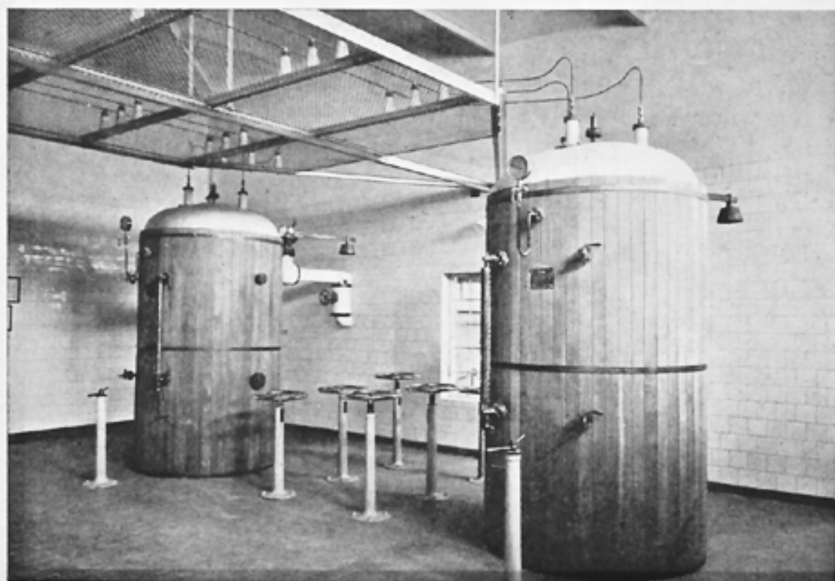
Aus der Zentralwäscherei (Elektrokessel im Schafräume)
